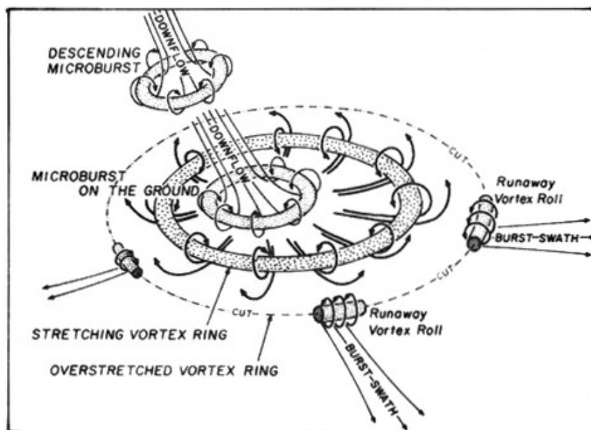
Fig. 2.3 – Ipotesi sulla genesi dei burst swaths (Fujita, 1983).
