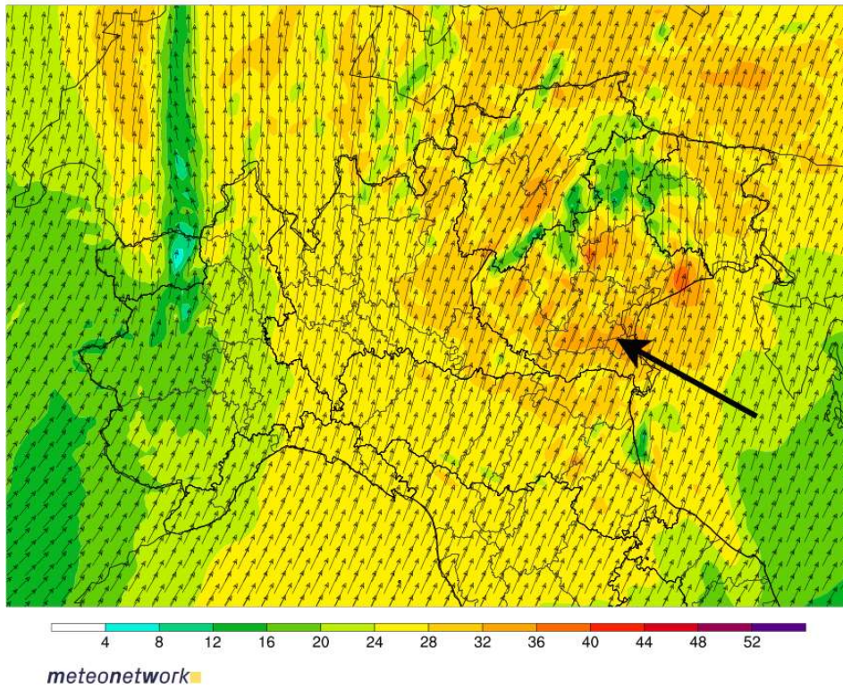
Fig. 4.36 - Venti a 500 hPa previsti dal WRF MeteoNetwork alle 13 UTC del 10 agosto 2017, Run 06 UTC.
