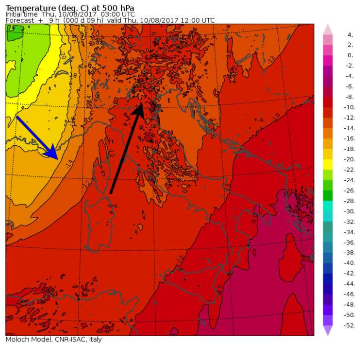
Fig. 4.21 - Temperature a 500 hPa previste dal modello Moloch il 10 agosto 2017 alle 12 UTC, Run 00 UTC.
