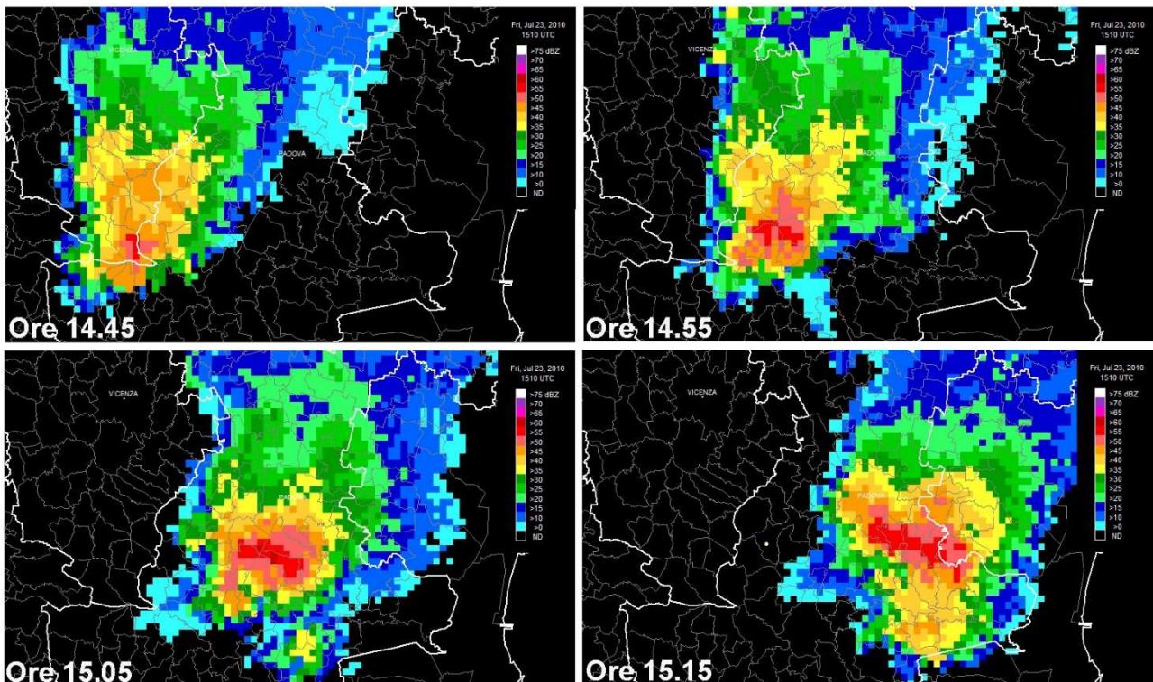
Fig. 5.21 – Immagine radar ARPAV/CMT di Concordia Sagittaria (VE) con riflettività massima (CMAX). Orari UTC.
