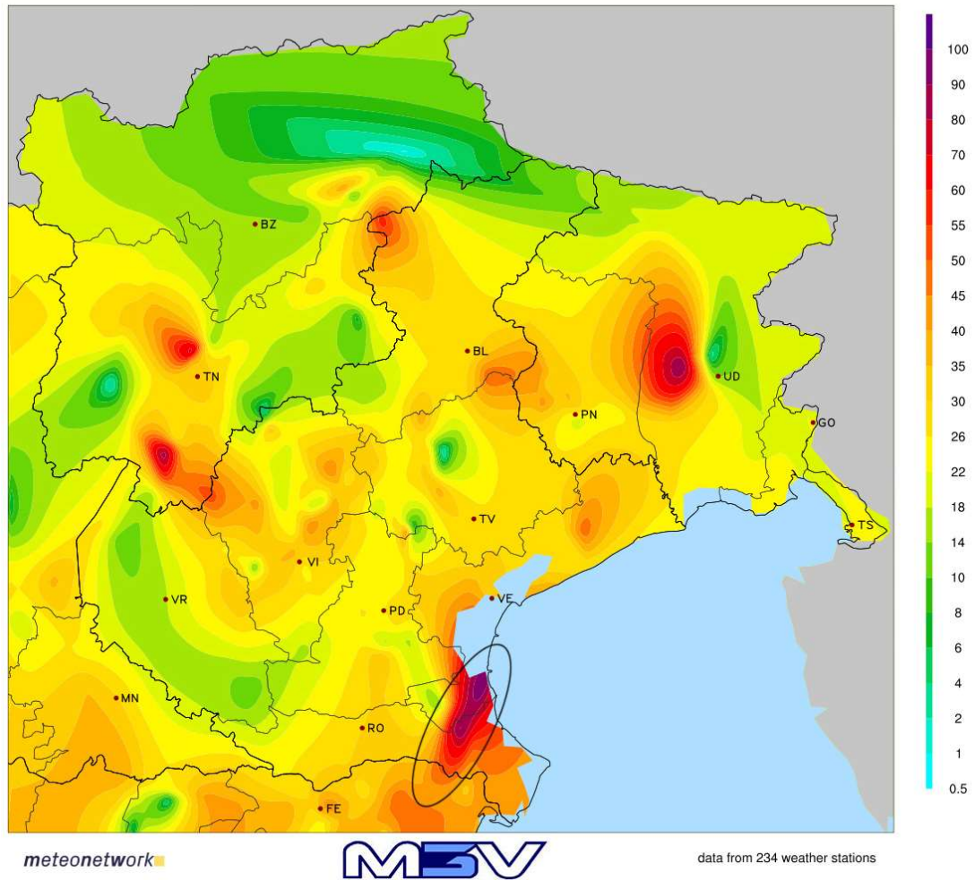
Fig. 5.71 – Raffica massima in km/h del 10 agosto 2017 tra Emilia Romagna, Veneto e Friuli Venezia Giulia delle stazioni della rete MeteoNetwork/MeteoTriveneto. L'ellisse nera individua la fascia di territorio colpita dai downbursts.
