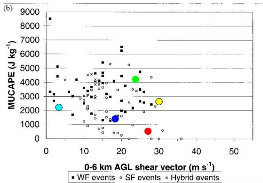
Fig. 4.58 - Relazione tra MUCAPE e shear 0-6 km. I pallini colorati rappresentano i casi studio: 12 UTC del 5 agosto 2016 (pallino rosso), 10 agosto 2017 (pallino verde), 23 luglio 2010 (pallino blu), 28 luglio 2006 (pallino celeste), 29 giugno 2006 (pallino giallo). Il pallino viola del 06 UTC del 5 agosto 2016 è assente in quanto il CAPE risultava negativo.
