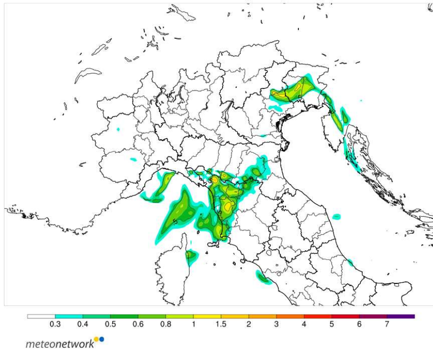
Fig. 4.12 - EHI previsto dal WRF MeteoNetwork il 5 agosto 2016 alle 9 UTC.
