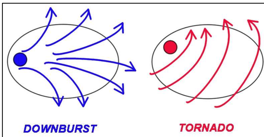
Fig. 3.2 – Simmetria dei danni da downburst e da tornado. Il cerchio blu rappresenta il punto di impatto del downburst, il cerchio rosso rappresenta il centro di bassa pressione del vortice.
