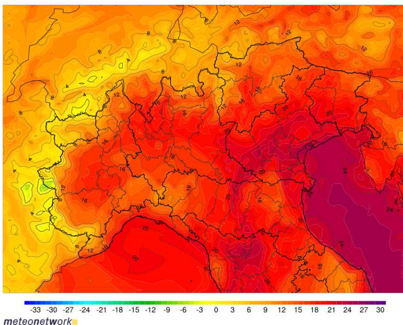
Fig. 4.30 – Dew points previsti dal modello WRF MeteoNetwork alle 12 UTC del 10 agosto 2017, Run 06 UTC.
