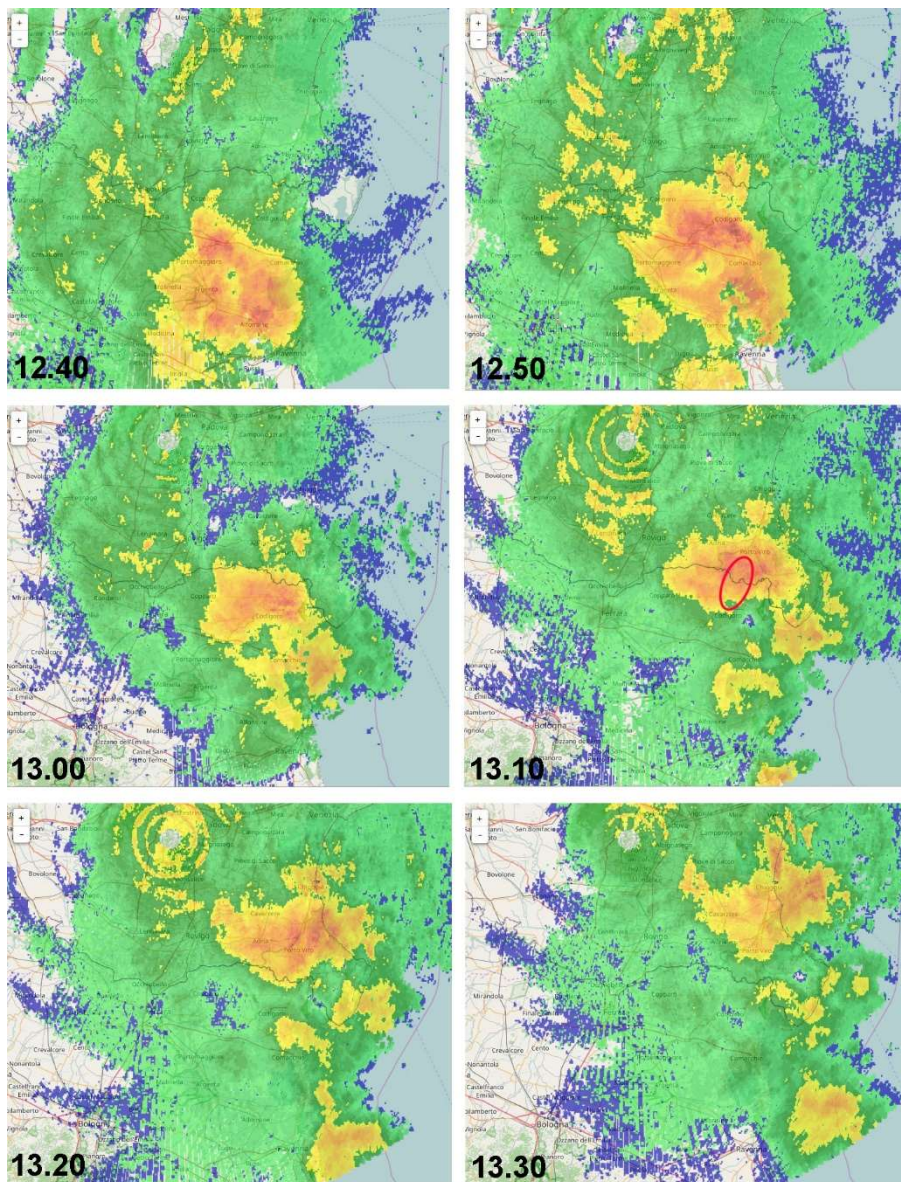
Fig. 5.68 – Immagini radar ARPAV/CMT di Teolo (PD) di riflettività massima, orari UTC. L'ellisse rossa indica l'area tra ferrarese e rodigino in cui si sono verificati i danni da downbursts, sovrapposta alla posizione del MCS.
