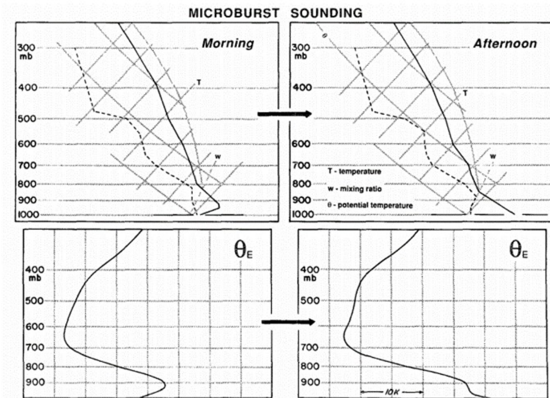
Fig. 4.48 - Grafici elaborati da Atkins e Wakimoto raffiguranti i profili favorevoli a microburst.
