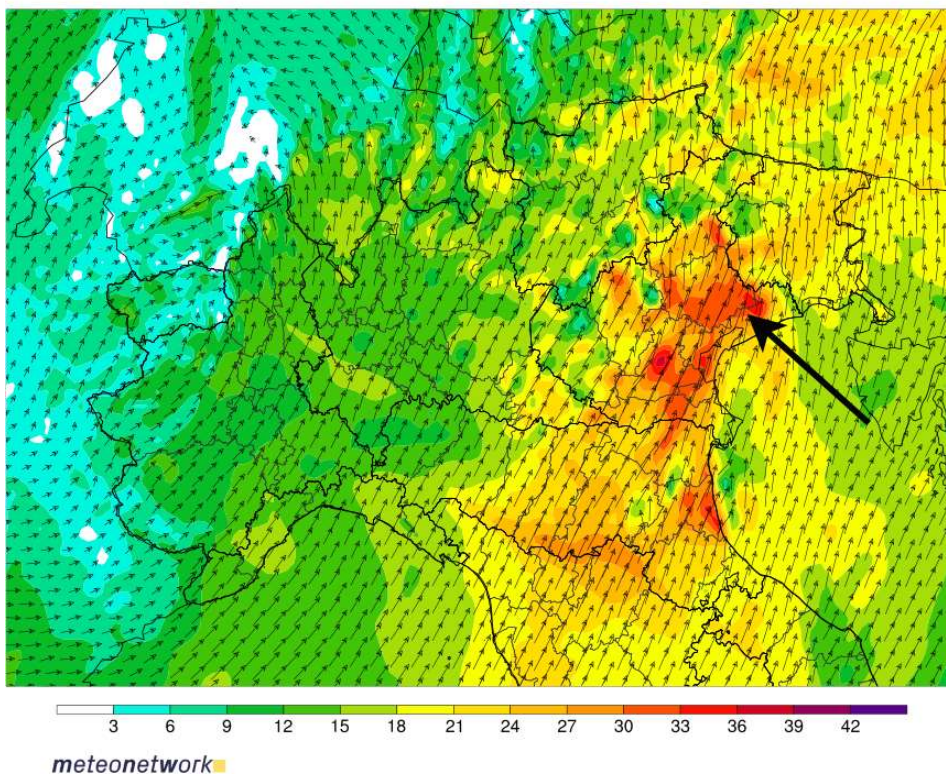
Fig. 4.37 - Venti a 700 hPa previsti dal modello WRF MeteoNetwork alle 13 UTC del 10 agosto 2017, Run 06 UTC.
