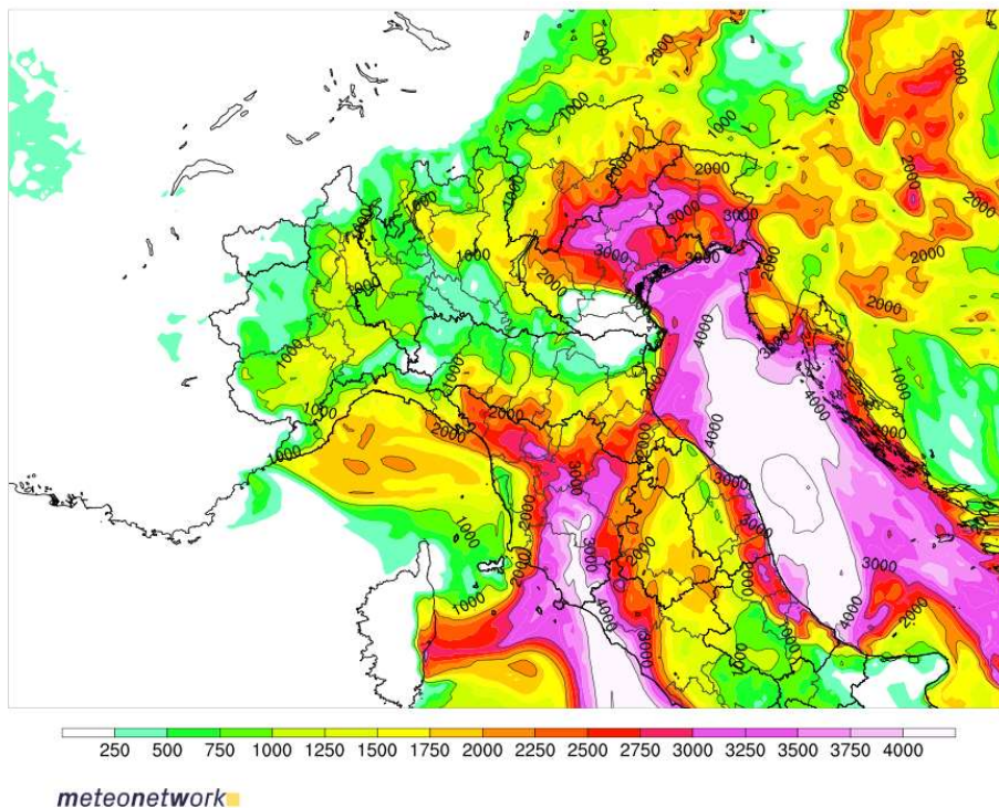
Fig. 4.31 - \mu CAPE previsto dal WRF MeteoNetwork alle 12 UTC del 10 agosto, Run 00 UTC.
