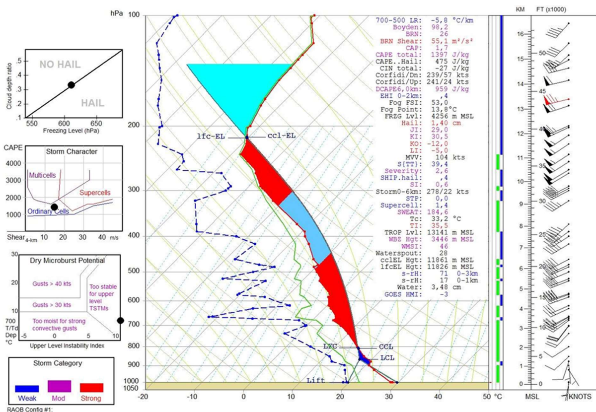
Fig. 4.59 - Radiosondaggio di Udine Campofornido del 23 luglio 2010 alle 12 UTC, elaborato con il software RAOB.
