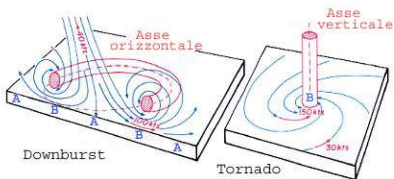
Fig. 3.1 – Schema dell'asse di rotazione nel downburst e nel tornado. Le velocità indicate sono rappresentative ed espresse in nodi, A e B denotano i campi di alta e bassa pressione al suolo generati dai due fenomeni in esame (Fujita, 1983).
