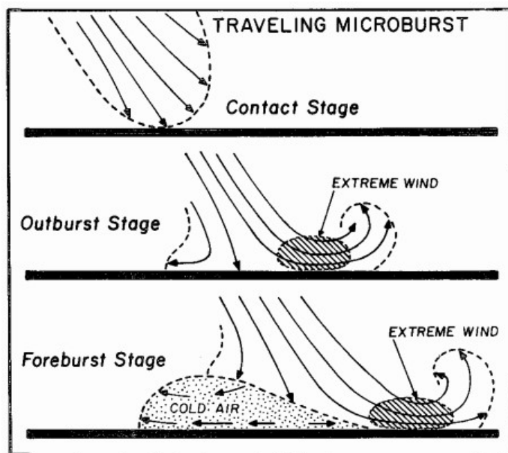
Fig. 2.1 – Schema evolutivo di un downburst in movimento verso destra (Fujita, 1981).
